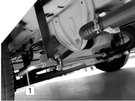
Kuva 83: Tyhjennysventtiilin tanko, esimerkki
